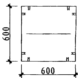
Q-BIC雨水箱侧视图
