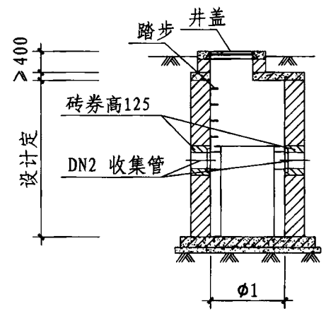
4-4剖面图 (做法II)
