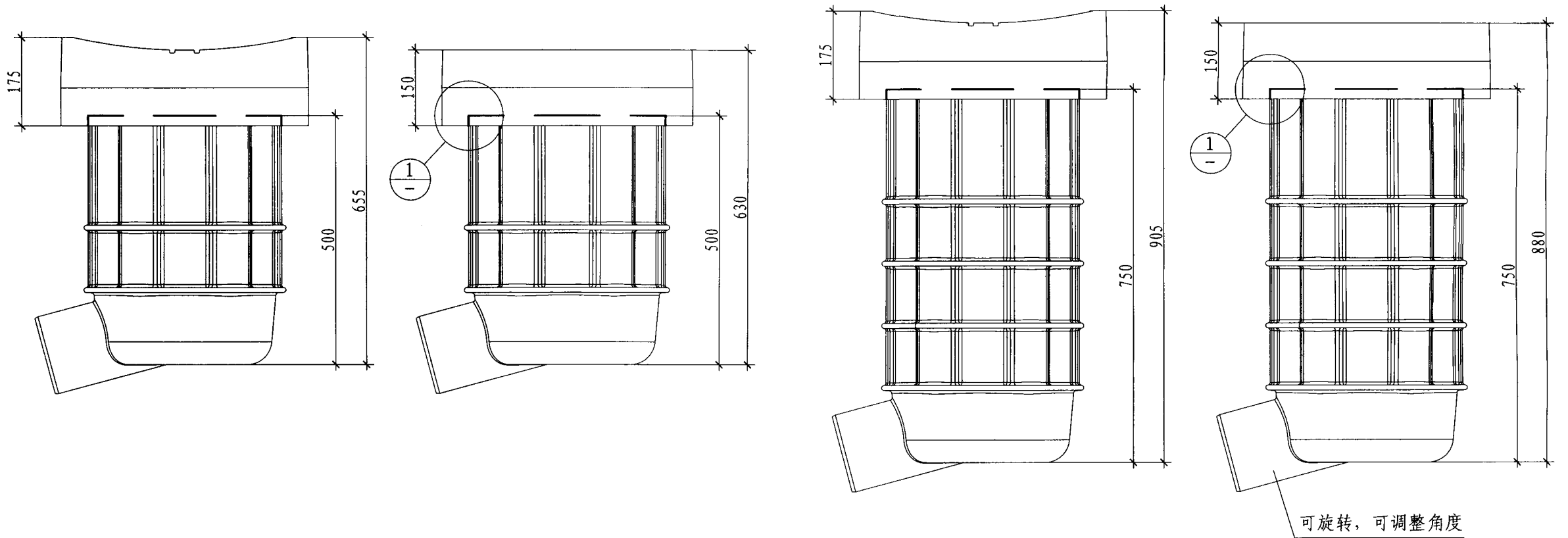
浅式 (KF) - 凹型拦污雨水口
