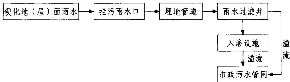
图2 埋地入渗系统的构成
