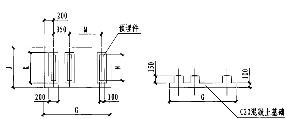
弃流控制器基础图
