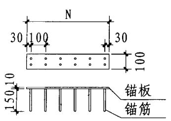
预埋件大样图
