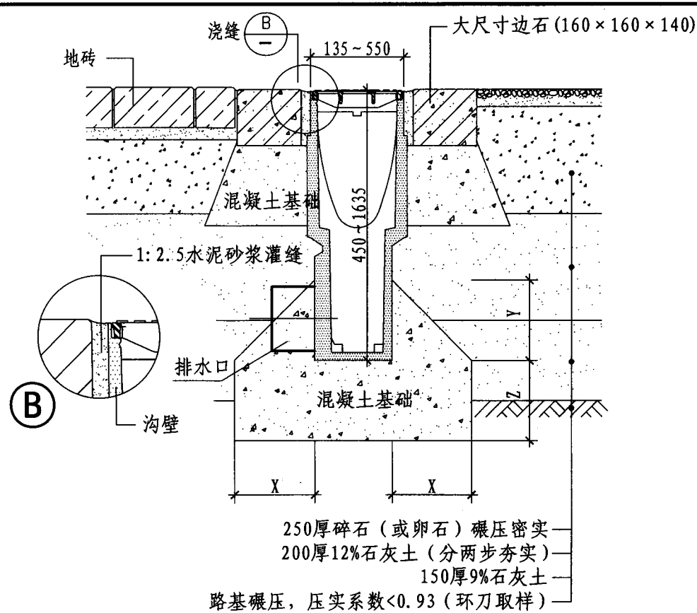
V型排水沟跌水井安装
