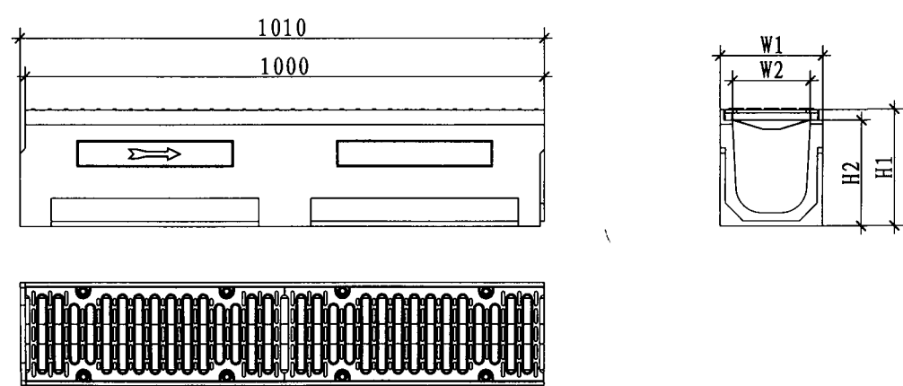
树脂混凝土排水沟大样图
