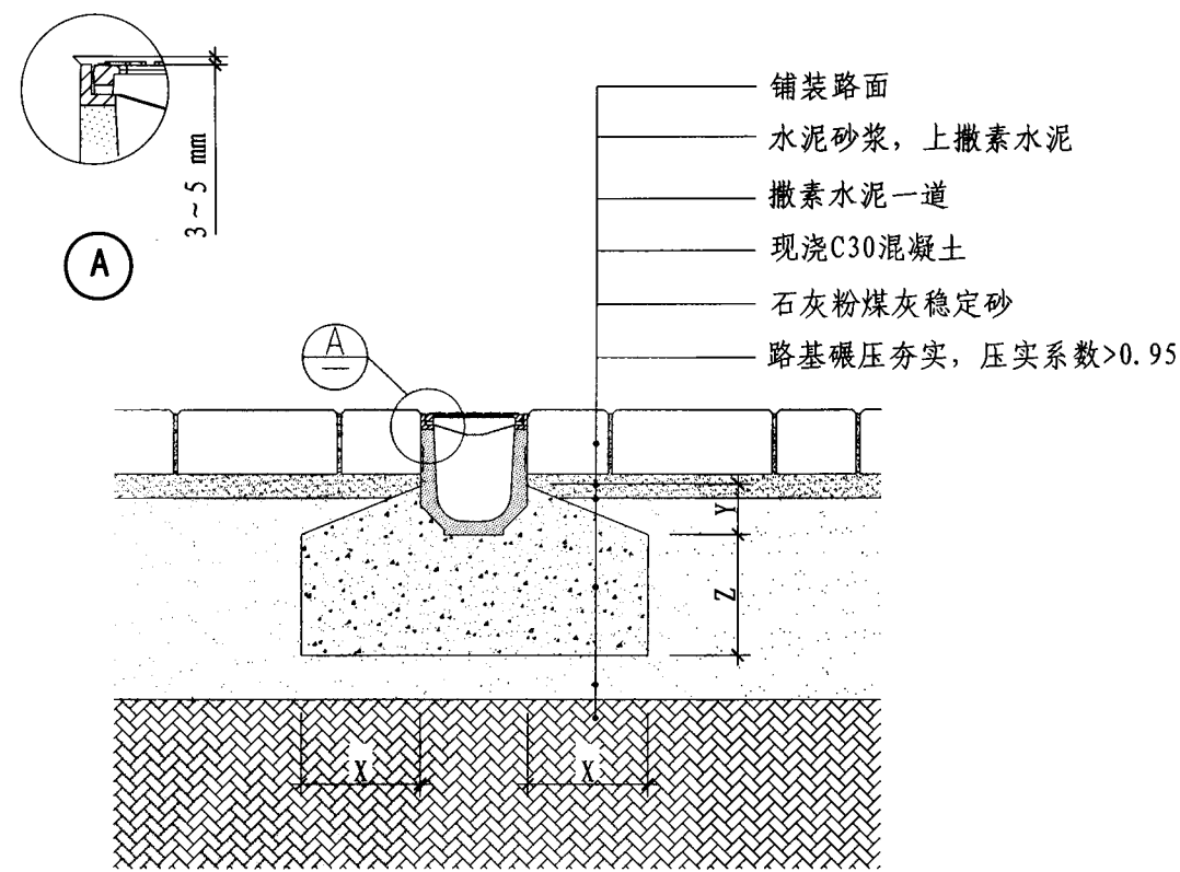
树脂混凝土排水沟安装图
