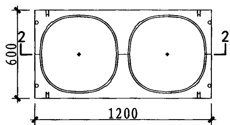
Q-BIC雨水箱立面图
