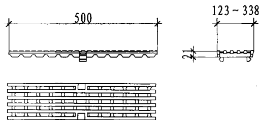
栅条盖板
