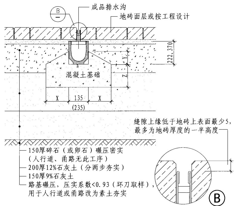
中缝式排水沟安装 沟净宽100 (200)
