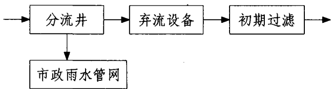
图6 弃流系统
