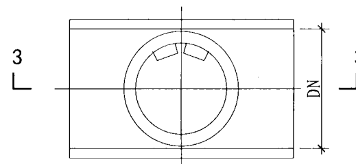
四通式检查井结构图
