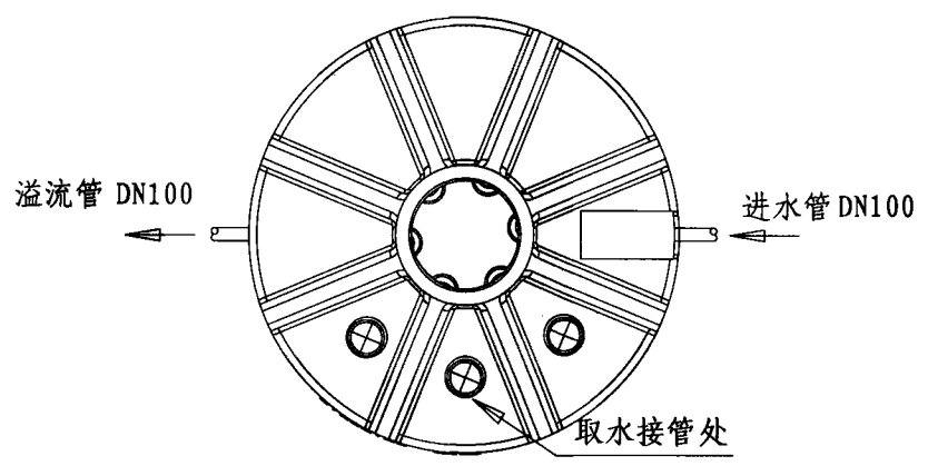
CG-3.5和CG-5.0储水罐
