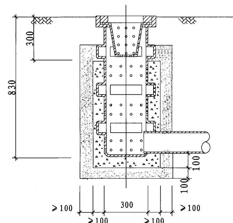
2-2剖面图
