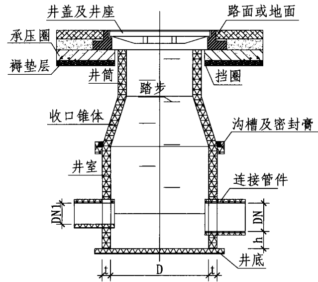
3-3剖面图
