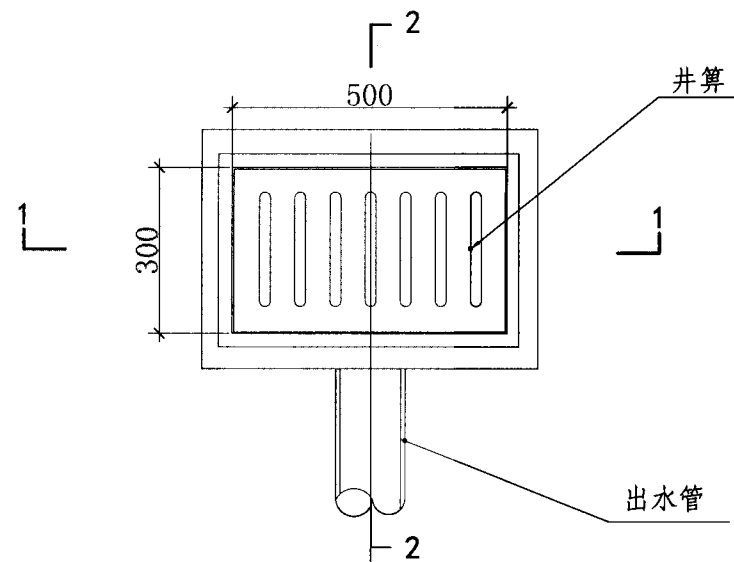
平面图
