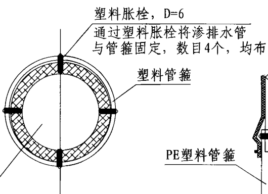
片材与管材连接大样（2）
