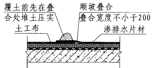
土工布的搭接
