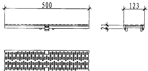
防鞋跟陷入盖板
