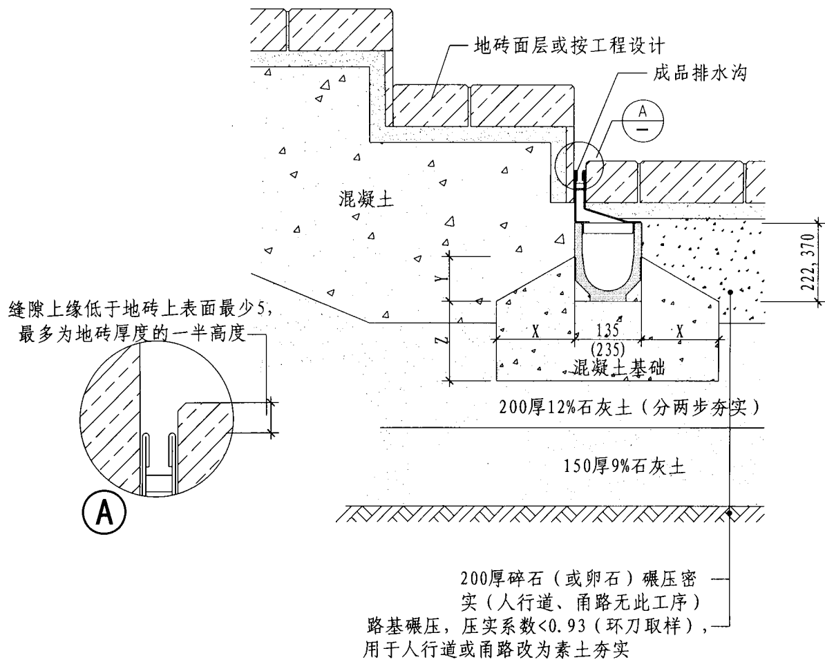
侧缝式排水沟安装 沟净宽100 (200)
